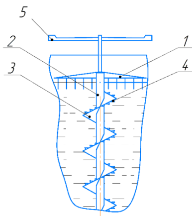
Рисунок 5- Схема модернизированного биореактора-метантенка ИБГУ-1 [1]: 1 - гребенка; 2 - вал мешалки; 3 - шнек; 4 - режущий сегмент; 5 - рукоятка-крестовина мешалки;
