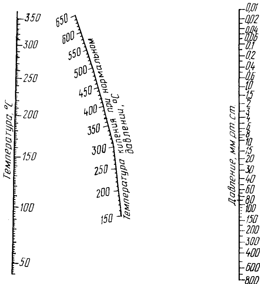
Рисунок 2- Номограмма ИОР
