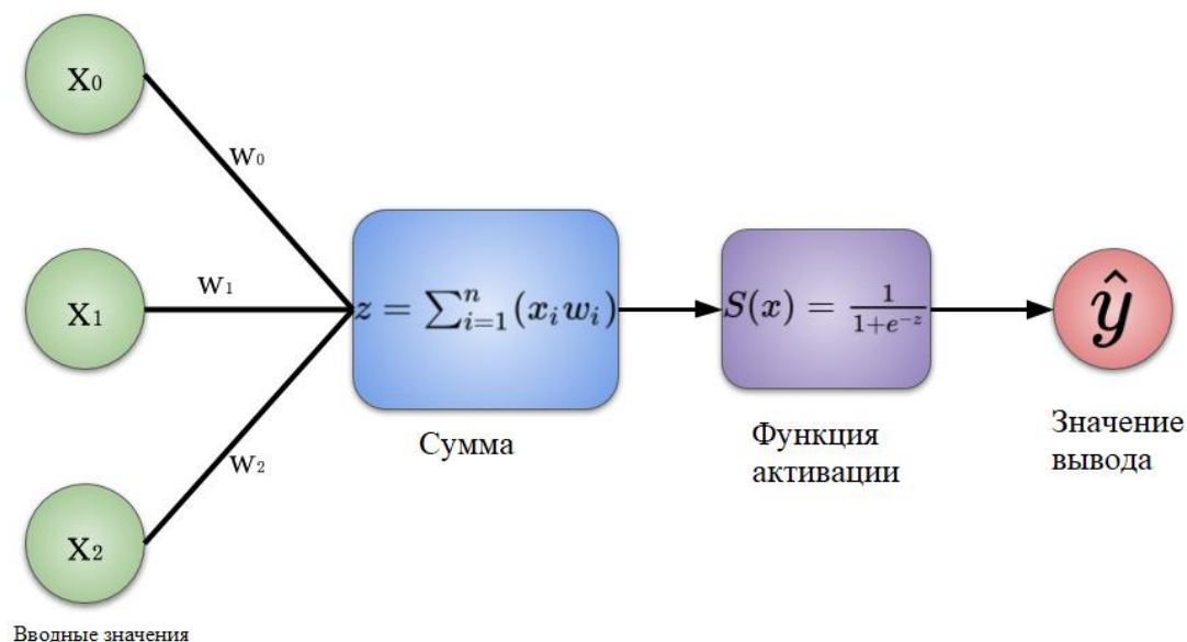
Рисунок 1 – Модель реализации нейронной сети
