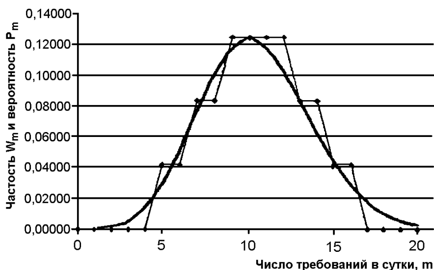
Рисунок 2 – График опытного распределения числа требований на ремонтно-обслуживающие работы и распределение Пуассона
