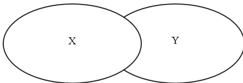
Рисунок 1 – Пересечение множеств X & Y
