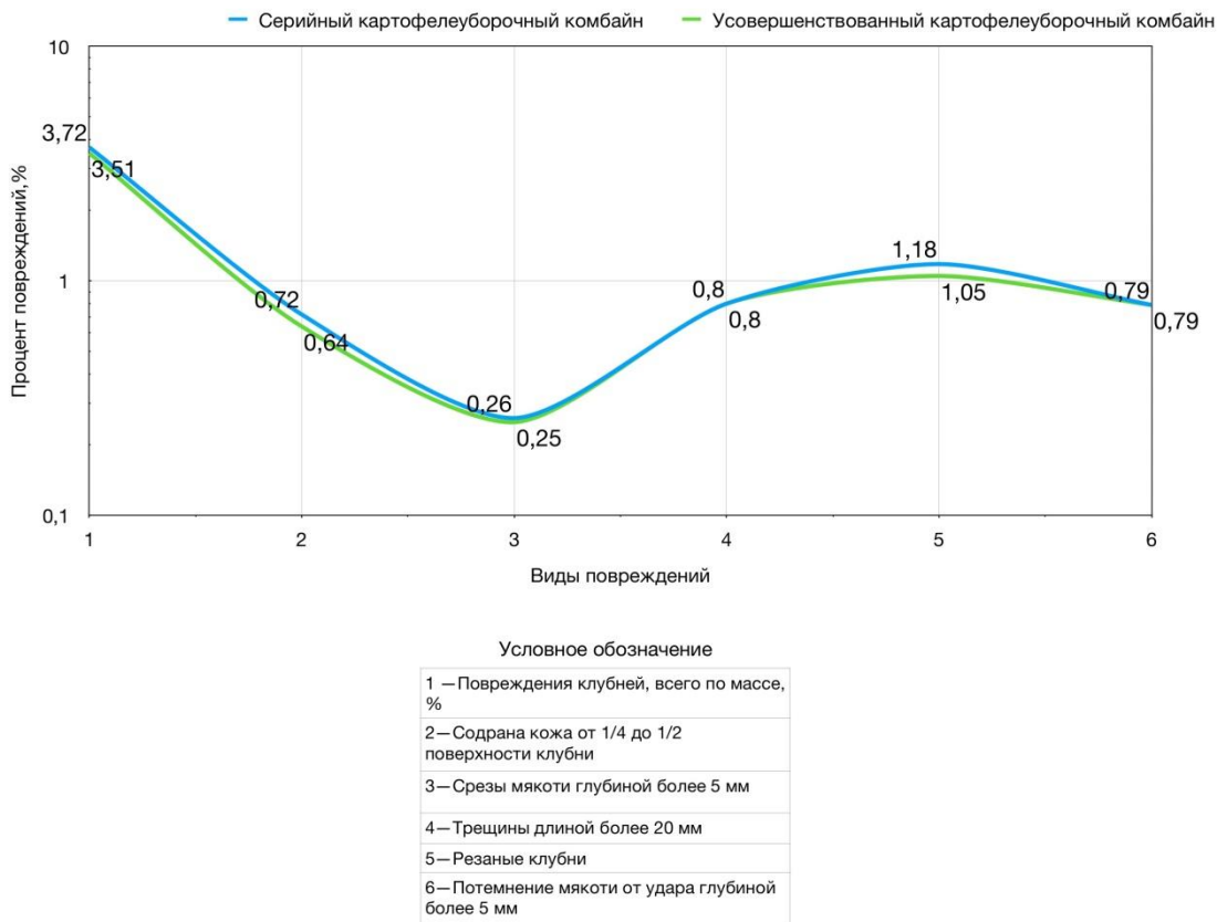
Рисунок 8. - Повреждения клубней в процентном соотношении при уборке картофеля двумя картофелеуборочными комбайнами
