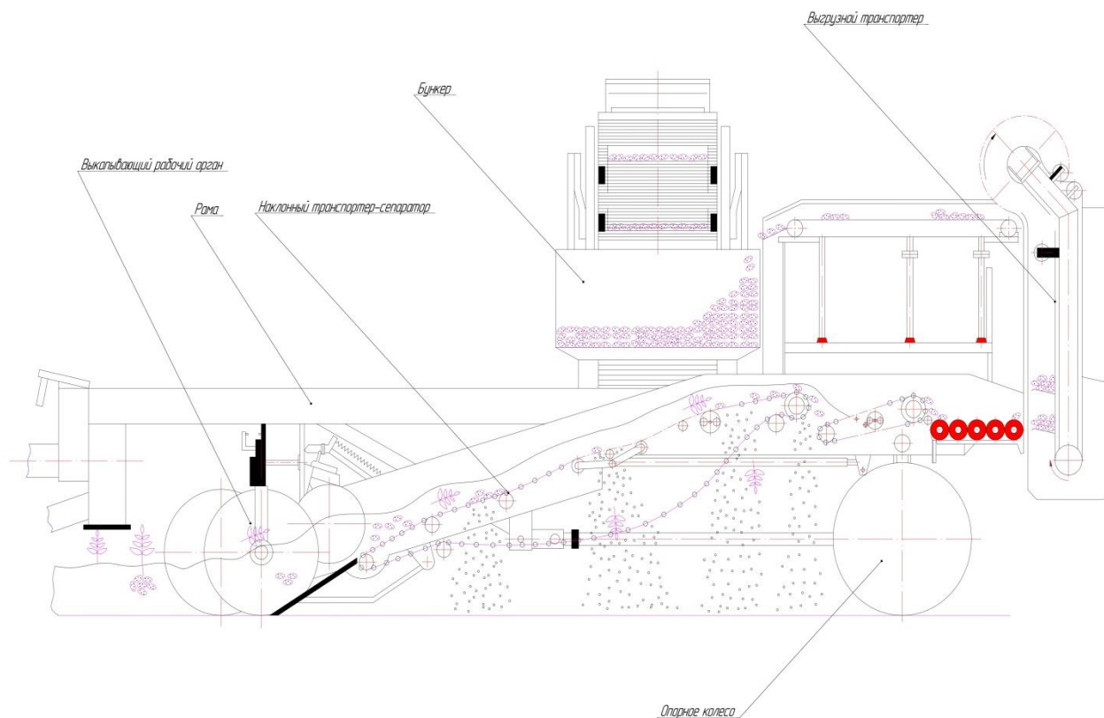
Рисунок 2. - Уборка картофеля картофелеуборочным комбайном
