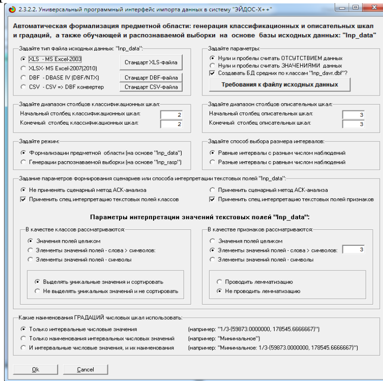
Рисунок 2. Экранная форма управления API-2.3.2.2
