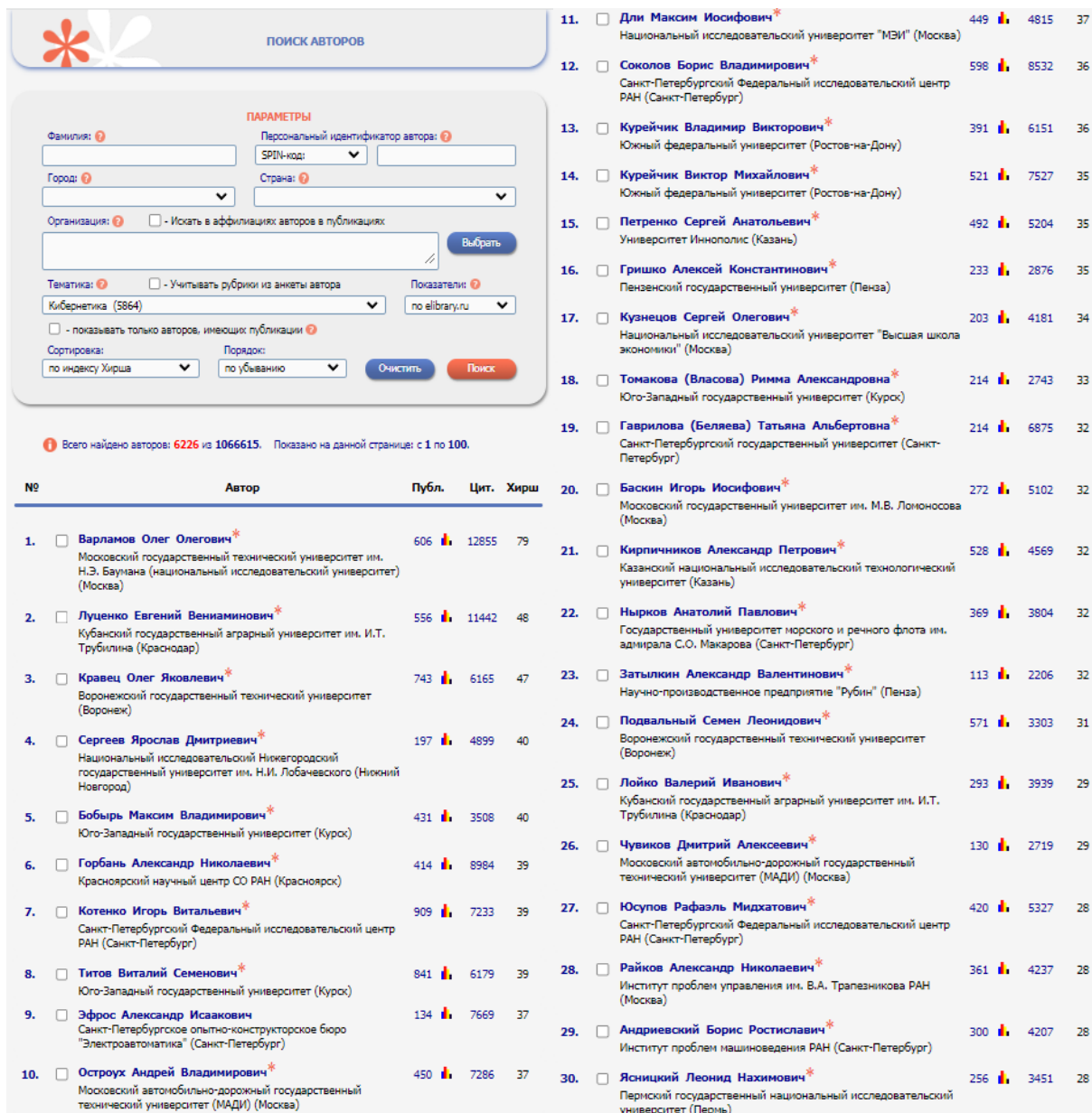
Рисунок 1. ТОП-30 российских ученых в области кибернетики (по индексу Хирша по данным РИНЦ)
