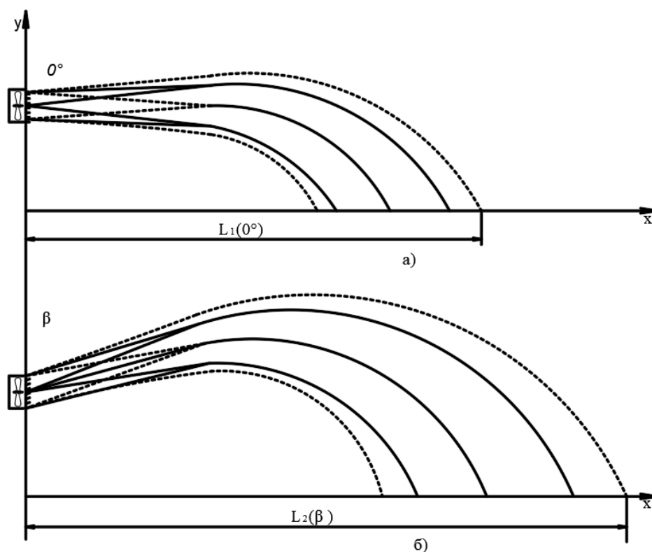
Рисунок 1 – Схема распространения охлажденной струи:
