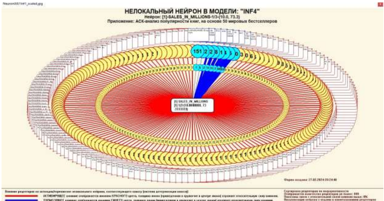
Рисунок 34 – Нелокальный нейрон, соответствующий классу SALES_IN_MILLIONS 1/3
