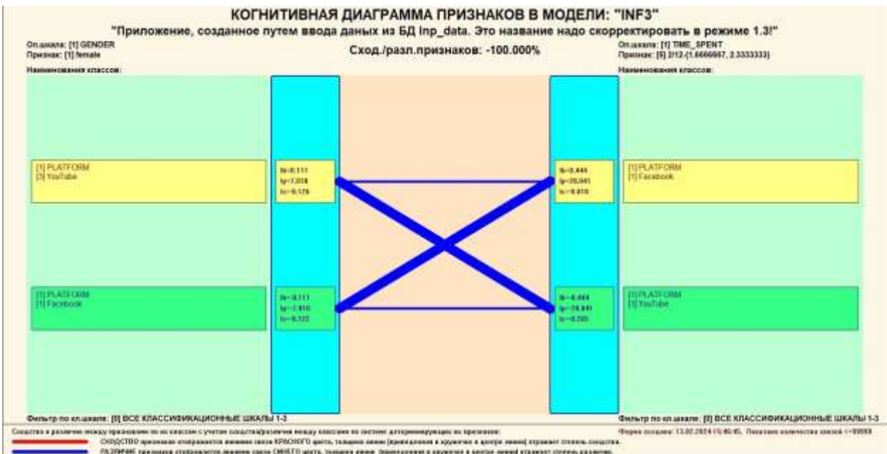
Рисунок 31. Примеры 2d-интегральных когнитивных карт содержательного сравнения значений факторов по их влиянию на переход объекта моделирования в состояния, соответствующие классам в СК-модели INF3
