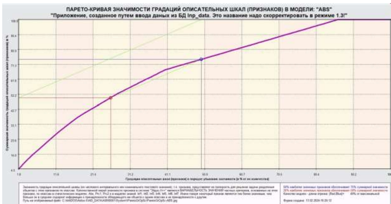
Рисунок 33. Парето-кривая силы влияния значений факторов на поведение объекта моделирования в СК-модели ABS
