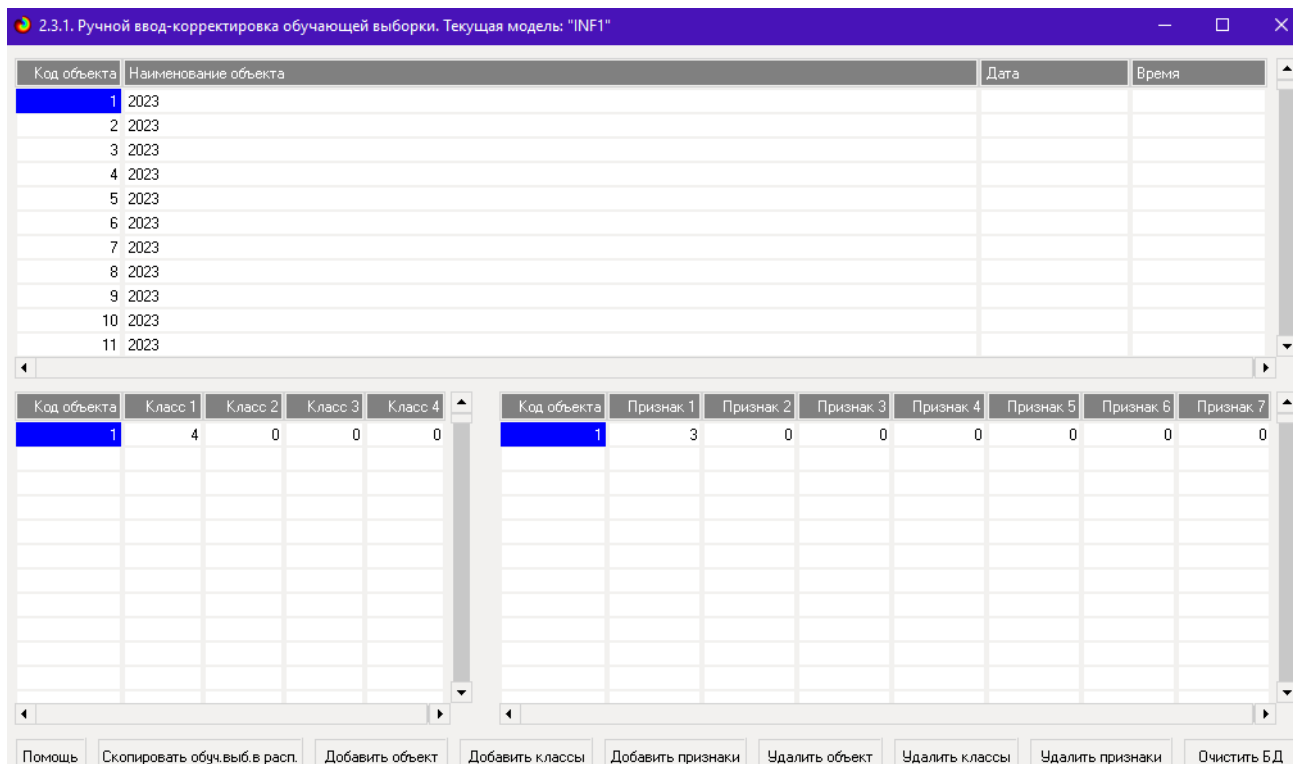
Рисунок 10 – Ручная корректировка
