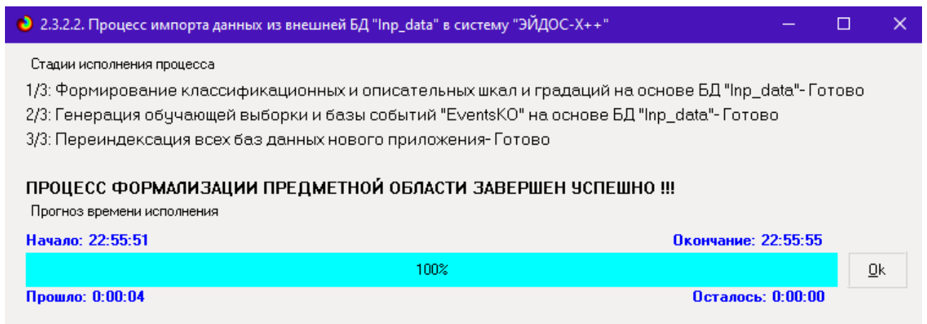
Рисунок 7 – Импорт данных
