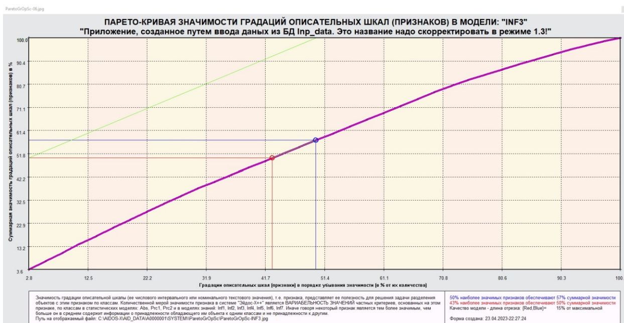
Рисунок 36 – Парето-кривая значимости градаций описательных шкал
