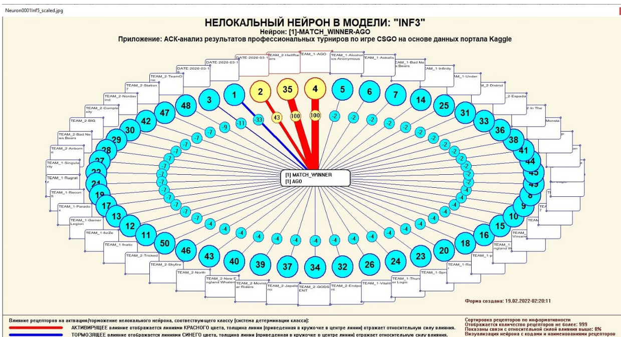
Рисунок 32 – Нелокальный нейрон в модели «INF3»
