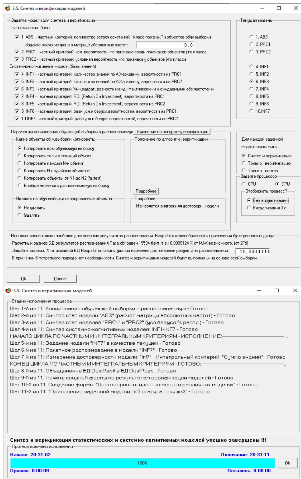
Рисунок 8. Экранные формы режима синтеза и верификации статистических и системно-когнитивных моделей системы «Эйдос» Обратим внимание на то, что на рисунке 8 в правом нижнем углу окна задана опция: «Расчеты проводить на графическом процессоре (GPU)».
