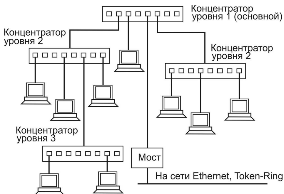
Рис. 63. Топология 100VG-AnyLAN
