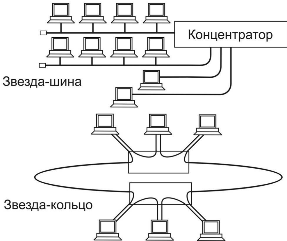
Рис. 51. Комбинированные топологии
