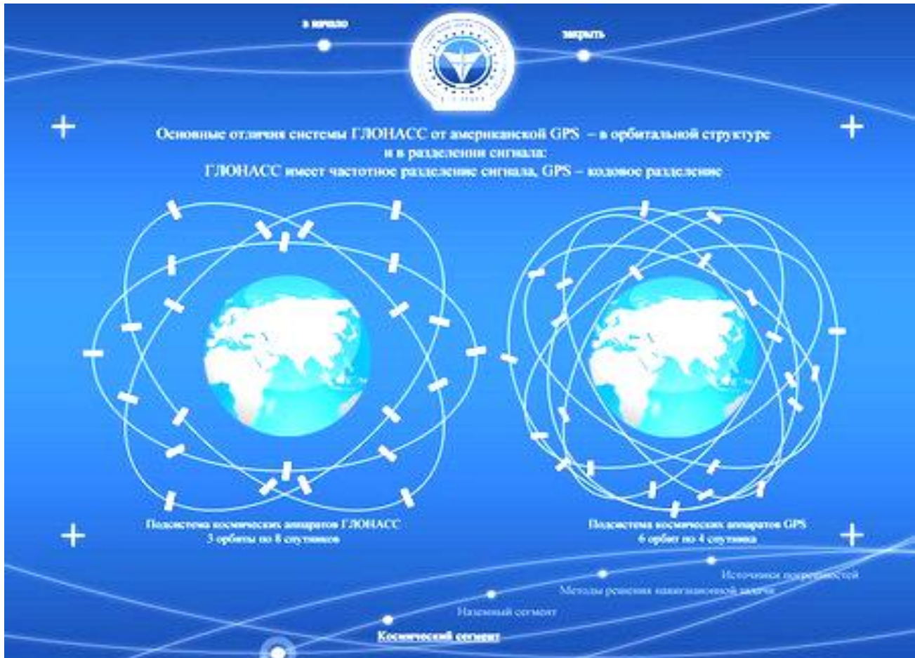
Рис. 101. Система ГЛОНАСС
